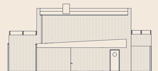
SEKTION C-C
