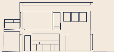
SEKTION B-B
