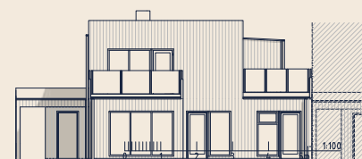
FASAD MOT NORDVÄST
