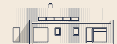
FASAD MOT SYDVÄST
