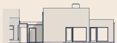
FASAD MOT NORDOST
