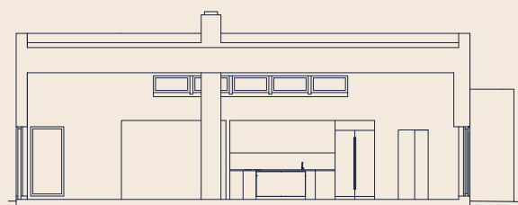
SEKTION H-H
